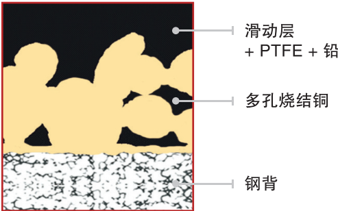
截面图
